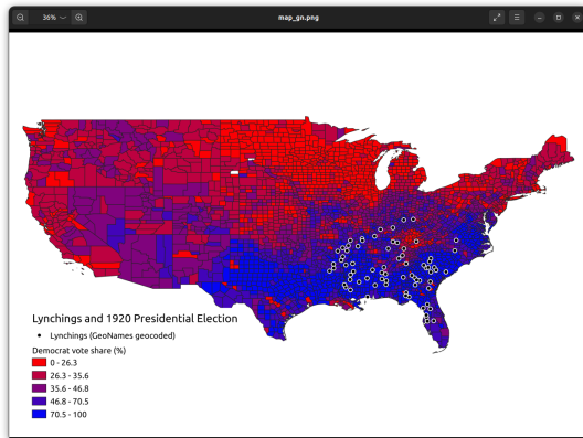
Figure 13: GeoNames map
