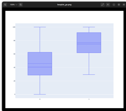
Figure 12: GeoNames boxplot
